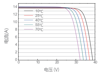
电流-电压曲线 JAM54S30-405/MR
